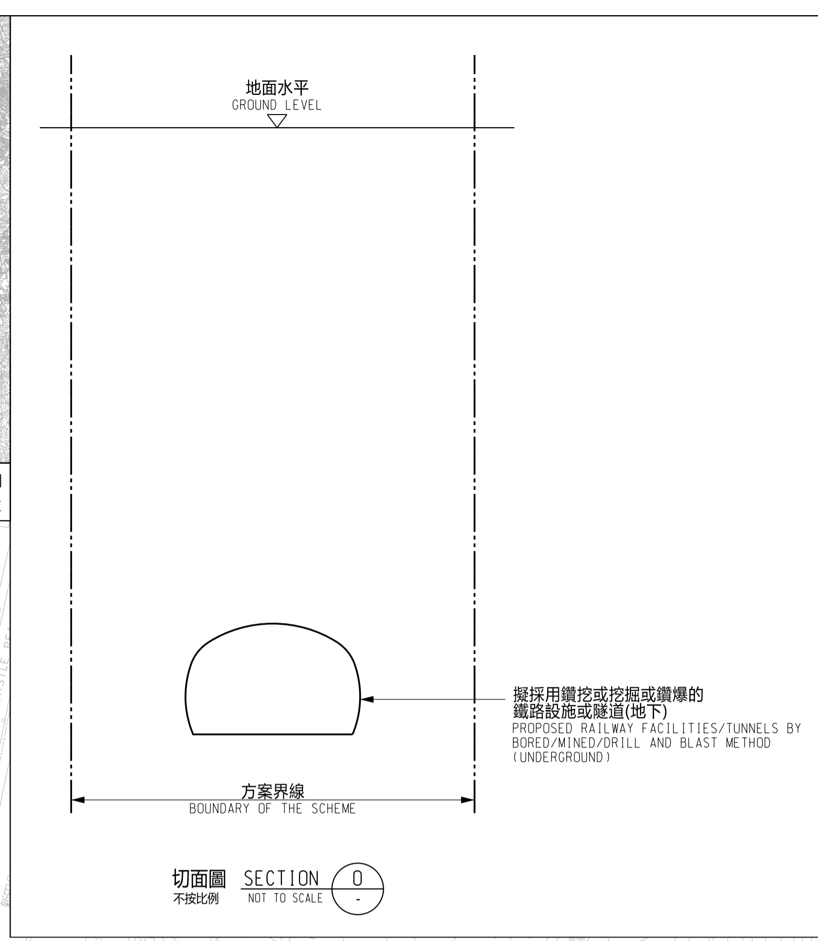
切面圖 SECTION 0 不按比例 NOT TO SCALE
